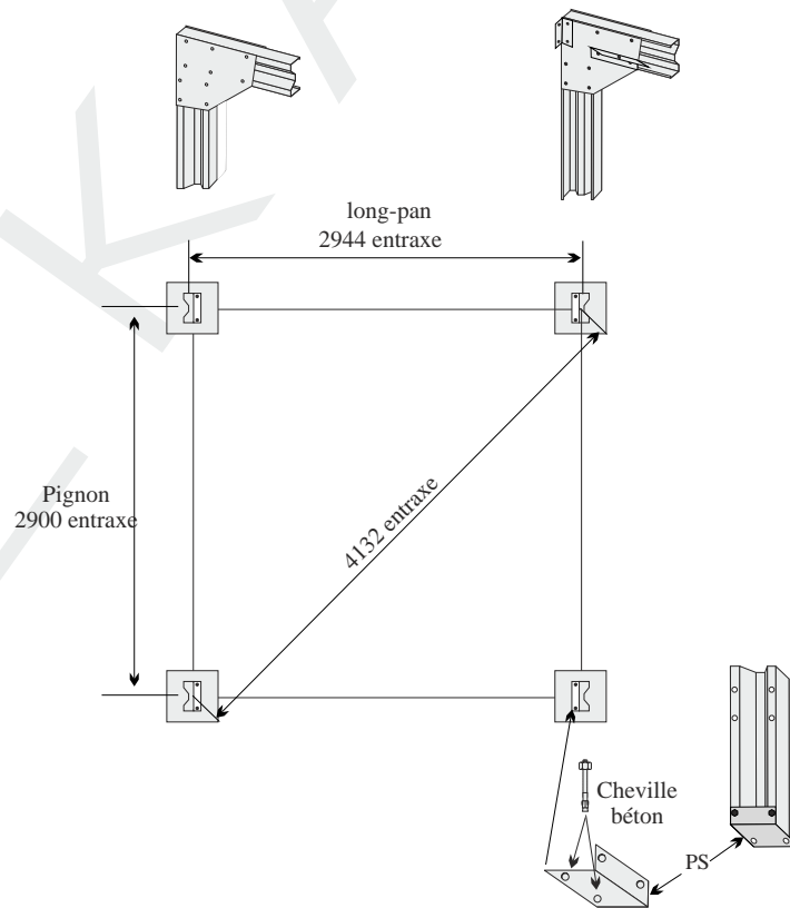
Plan et dimensionnement des plots béton et de la semelle pour un ECO33 positionnement des pannes sur les plots et liaison des platines au béton
